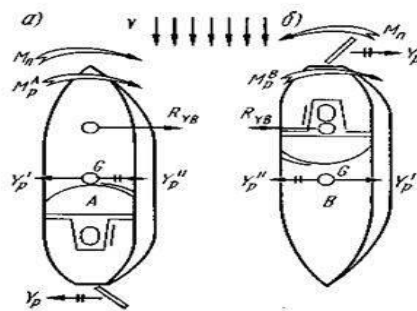
Рис. 14.8. К анализу причин плохой управляемости судна на заднем ходу
