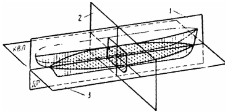
Рис. 35. Основные плоскости проекций теоретического чертежа: 1 — диаметральной плоскости, 2 — плоскости мидель-шпангоута, 3 — плоскости конструктивной ватерлинии
