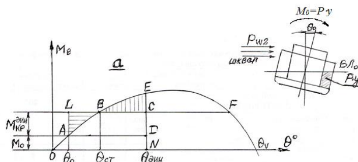
а) динамическое накренение судна с начальным креном \theta_0 от M_{\text{кр}} шквала P_{w2}
