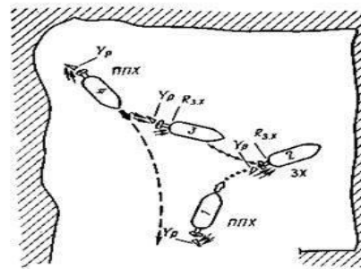
Рис. 14.9. Маневрирование судна на ограниченной акватории: ППХ — полный передний ход; ЗХ — задний ход
