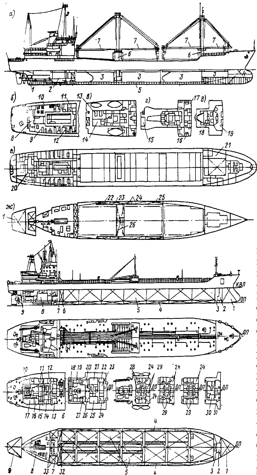
Рис. 83. Общее расположение помещений на танкере.
