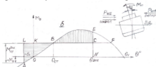
б) динамическое накренение судна с ветровым креном -\theta_0 от M_{\text{кр}} шквала P_{w2}
