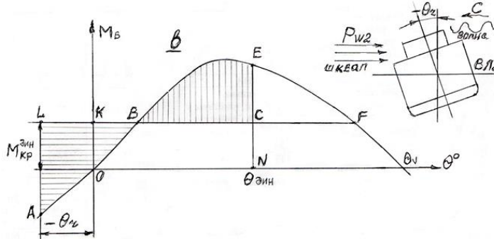
в) динамическое накренение судна с амплитудой качки -\theta_r от M_{\text{кр}} шквала P_{w2}
