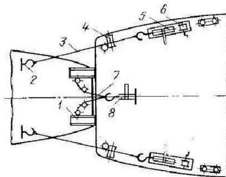
Схема двухупорного сцепного устройства.
