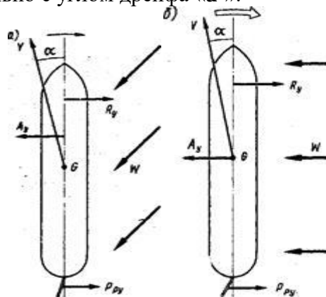
Рис. 9.4. Силы и моменты, действующие на судно в зависимости от курсового угла кажущегося ветра:
